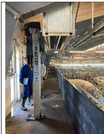
Figur 5. Klovbeskæringsboks på gangen mellem løbesti og drægtighedsstalden i besætning 2.
